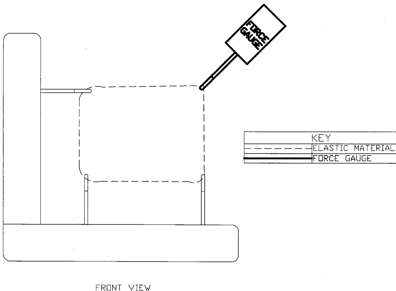
FIG. 346 (d) Test Procedure for Cords and Loops, Step 4 (continued)
