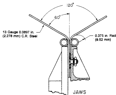
FIG.-28 30 Flexure Tester
